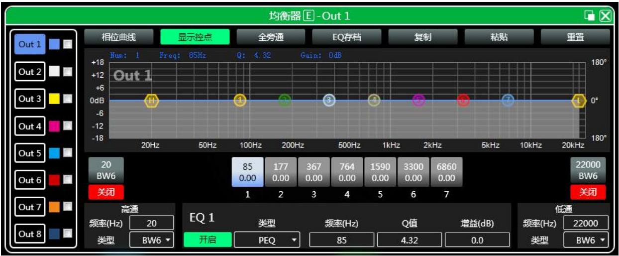
图 8.1 输出均衡器功能界面
