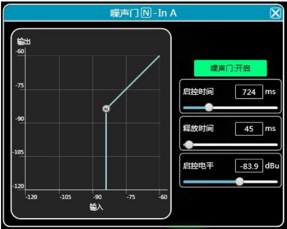
图 4.1 输入噪声门设置模块
